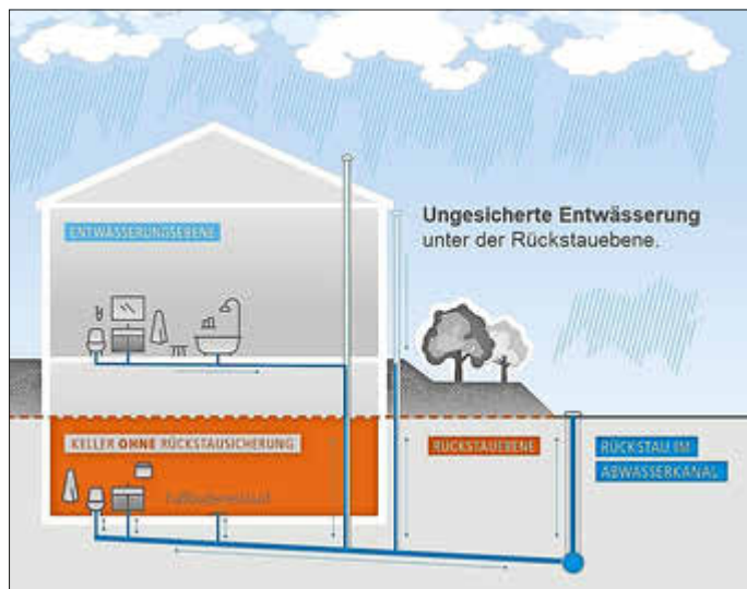
Abbildung: Darstellung einer Hausentwässerung bei Rückstau ohne Rückstausicherung Foto: Wasserwerke Zwickau
